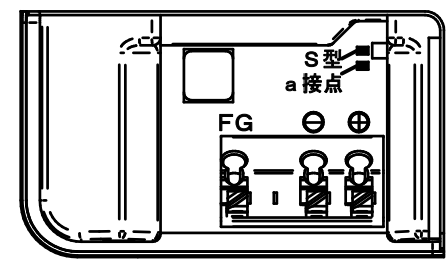
(端子部)
